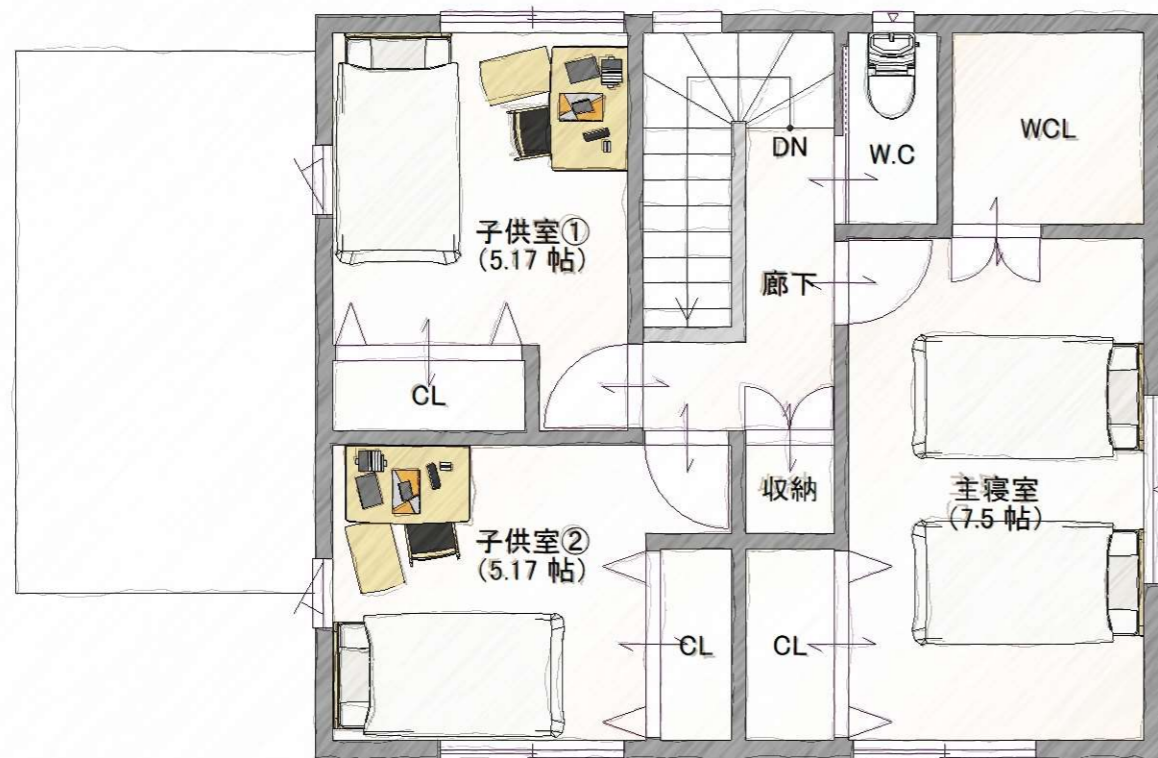
2階平面図 [ 1:100 ]
