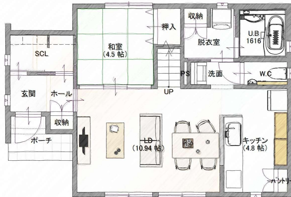
1階平面図 [ 1:100 ]
